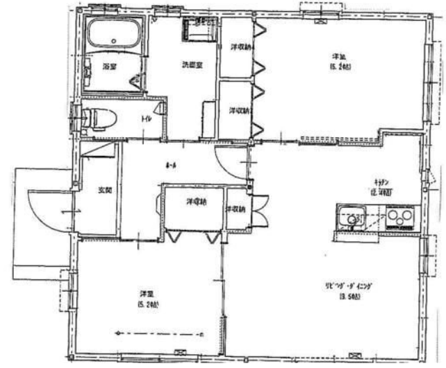
【間取り図】
