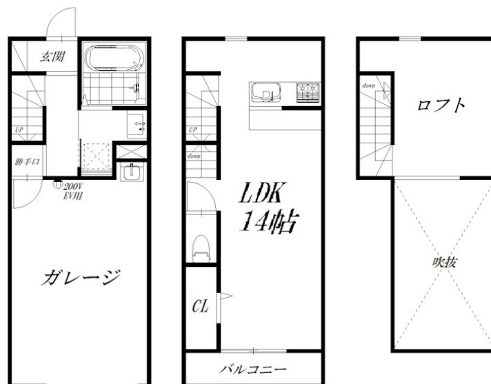
【間取り図】
