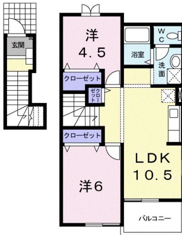
【間取り図】
